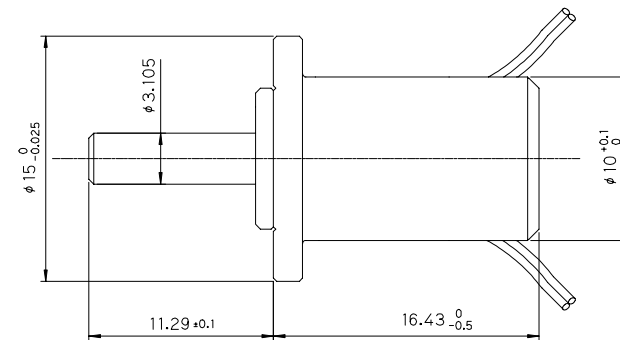
Dimension : mm
