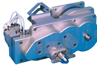
JEM用ストラクチャル ラッチアクチュエータ ACTUATOR- STRUCTURAL LATCH (JEM)
