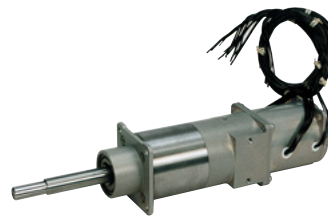
SFU用太陽電池フレキシブル パドル駆動用ACサーボモータ AC SERVO MOTOR (SFU)
